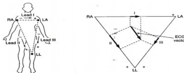
Fig.2.4 Einthoven Triangle
