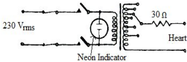
Fig.3.6 AC Defibrillator
