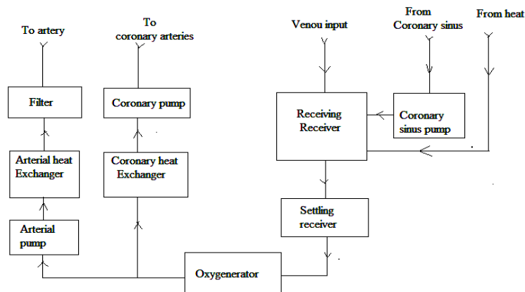
Fig.3.8 Heart Lung Machine
