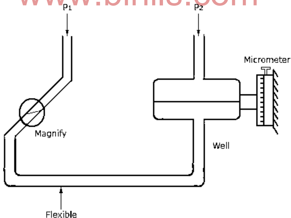
Micromanometer Fig.4.9
